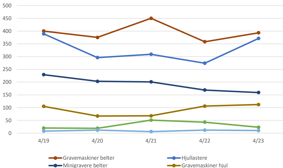
Fig. 1 – Viser utviklingen for 4. kvartal i 2019 – 2023 for de største undergruppene av anleggsmaskinstatistikken.
