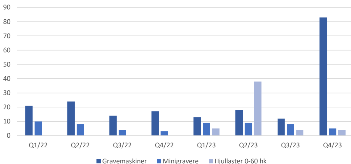
Fig. 3 – Viser antall nullutslippsmaskiner per kvartal siden 2022fordelingen for salg av gravemaskiner på belter fordelt på vektklasser for fjerde kvartal 2023. Klasser med færre en 10 solgte maskiner er ikke tatt med*
