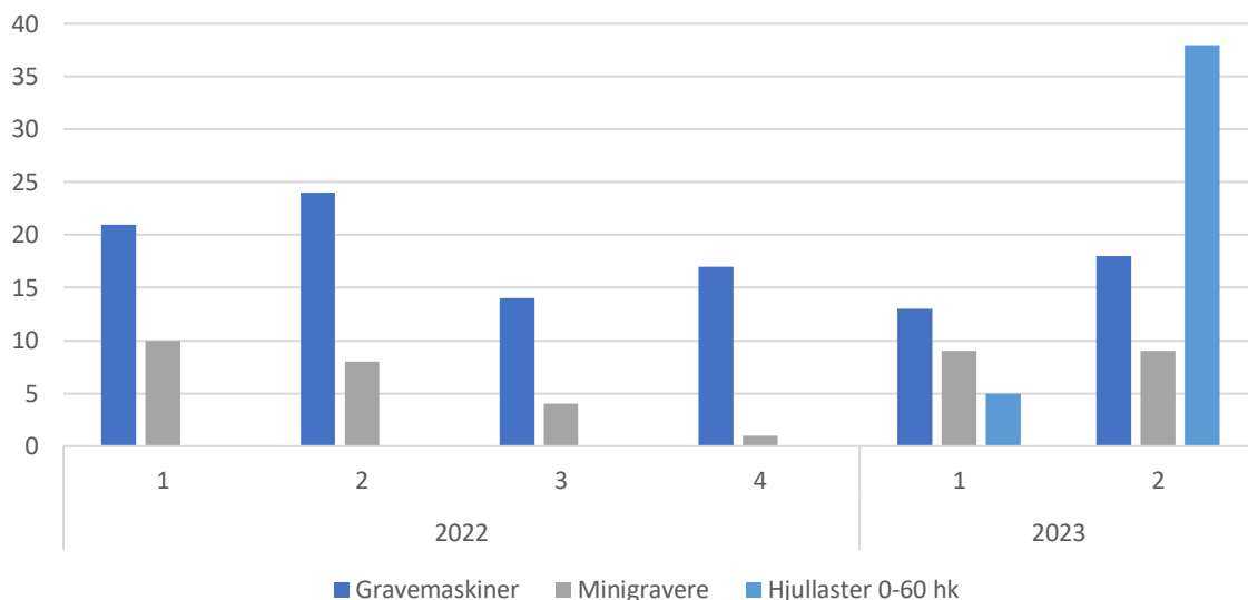
Fig. 3 – viser utviklingen i salg av nullutslippsmaskiner. NB! Hjullastere >60hk er med for første gang fra dette kvartalet
